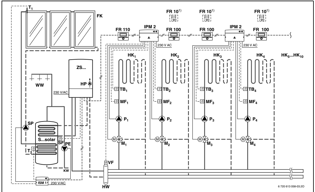
Bild 4 FR 110 und Heizgerät mit Speicheranschluss: Vereinfachtes Anlagenschema (montagegerechte Darstellung und weitere Möglichkeiten in den Planungsunterlagen)
