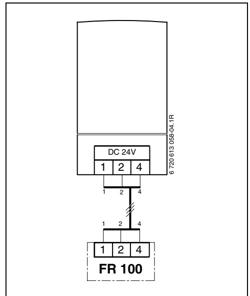
Bild 11 FR 100 über die analoge 1-2-4-Schnittstelle angeschlossen.
