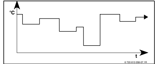
Bild 13 Beispiel Zeit-/Temperaturniveauprofil mit beliebigen Temperaturen für Heizprogramm D bis F
